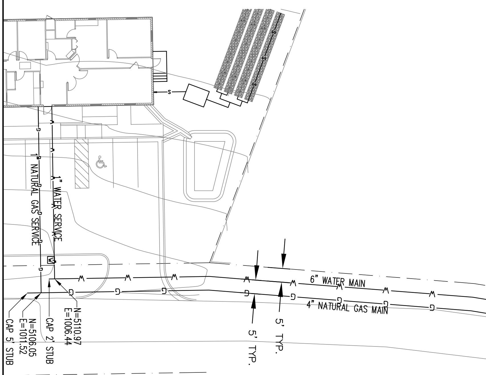
PLAN SCALE: 1" = 30'
